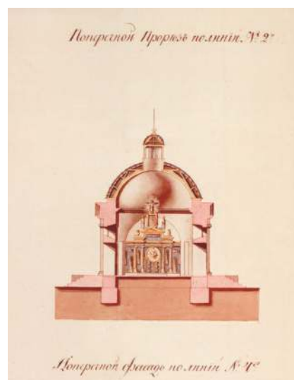
Рисунок 8. План каменной во имя святого Александра Невского Соборной церкви в Азовской крепости постройки 1803–1806 годов. Лист 2 [96]
