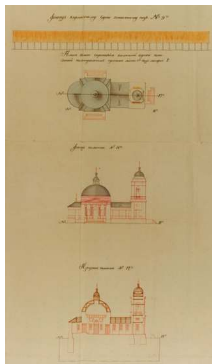
Рисунок 10. Чертеж увеличенных планов, фасадов и прорезей Александро-Невской церкви, состоящей в Азовской крепости... 1805 год [4]
